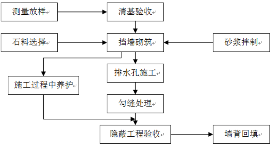
浆砌石挡土墙砌筑施工工艺流程图
