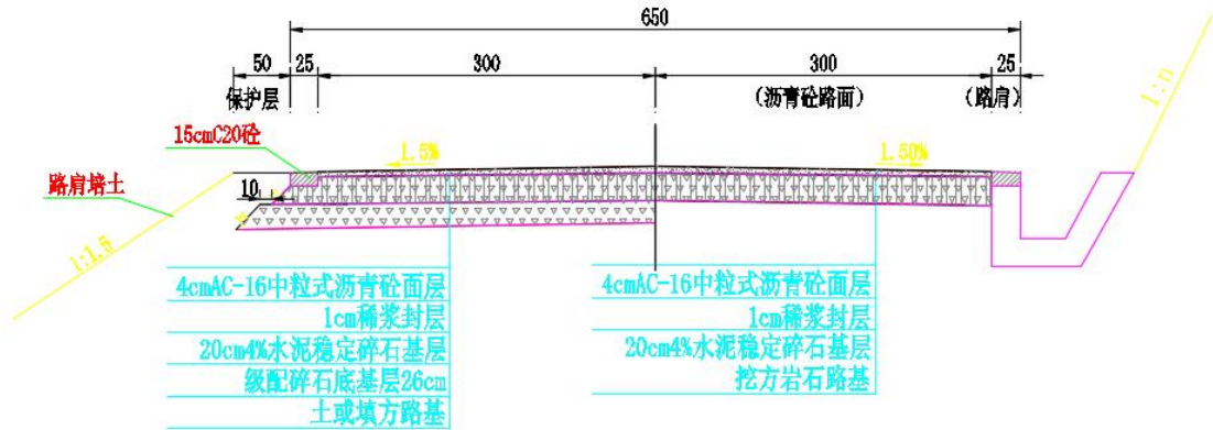
路面结构示意图
