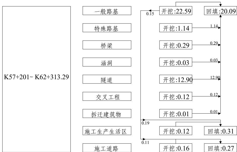
土石方流向框图(单位: 万 m³)
