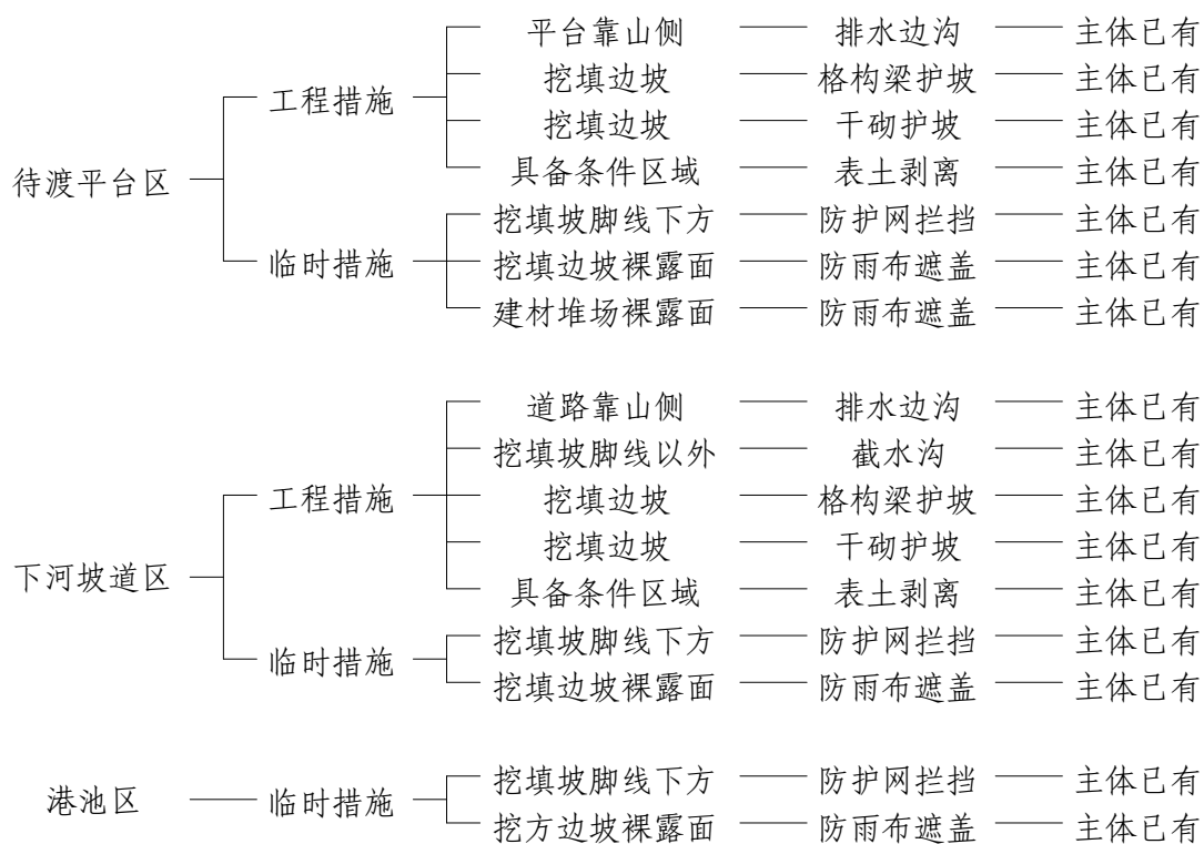
水土流失防治措施体系框图
