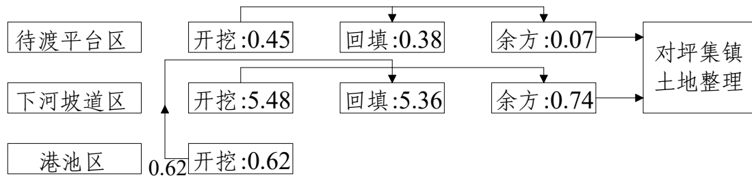
土石方流向框图(单位: 万 m³)
