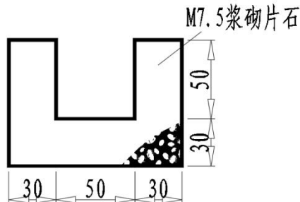
排水边沟标准断面图
