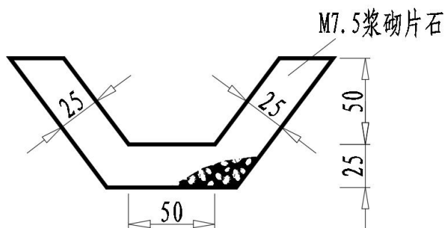
截水沟标准断面图
